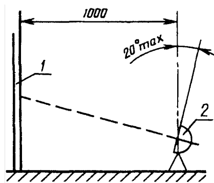
1 - радиометр; 2 - электрокамин
