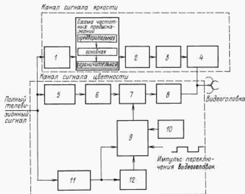
1 — фильтр сигнала яркости; 2 — частотный модулятор; 3 — фильтр верхних частот; 4 — усилитель записи; 5 — фильтр сигнала цветности; 6 — схема частотных предискажений плюс сигнал цветовой синхронизации, плюс 6 дБ; 7 — преобразователь частоты; 8 — фильтр нижних частот; 9 — преобразователь частоты и регистр сдвига; 10 — гетеродин; 11 — схема выделения сигналов строчной синхронизации; 12 — умножитель.
