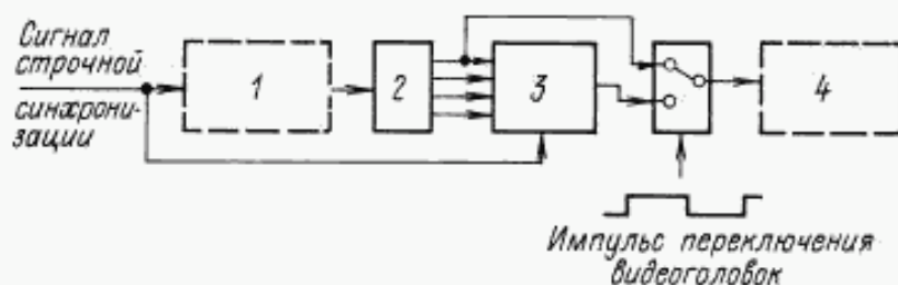
1 — умножитель частоты; 2 — делитель частоты на четыре; 3 — регистр сдвига фазы на 90^\circ ; 4 — преобразователь частоты
